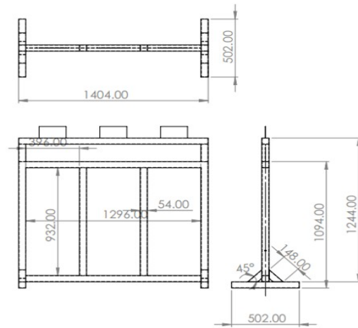
Gambar 2. Rangka tong sampah
