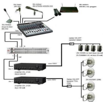
Gambar 1 Rangkaian input sound sistem
