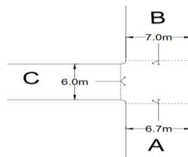
Gambar 3. Geometrik simpang
