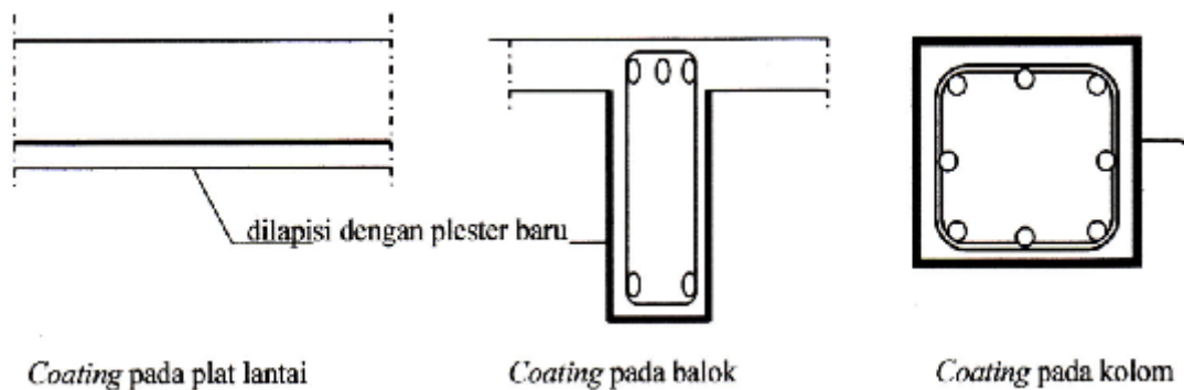
Gambar 2 : Coating pada plat lantai, balok dan kolom
