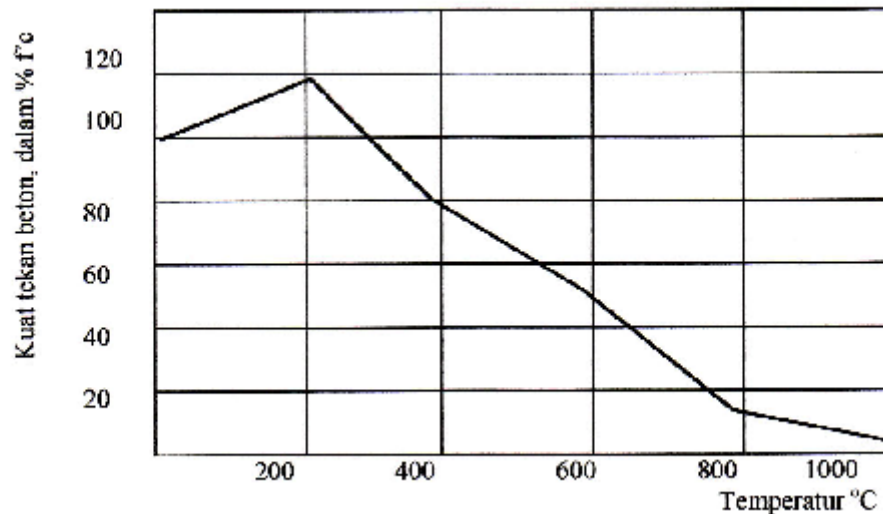
Gambar 1. Penurunan Kuat tekan beton Dalam Berbagai temperatur ( Suhendro 2000)
