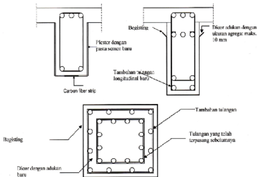
Gambar 4 : Prepacked concrete pada balok dan kolom
