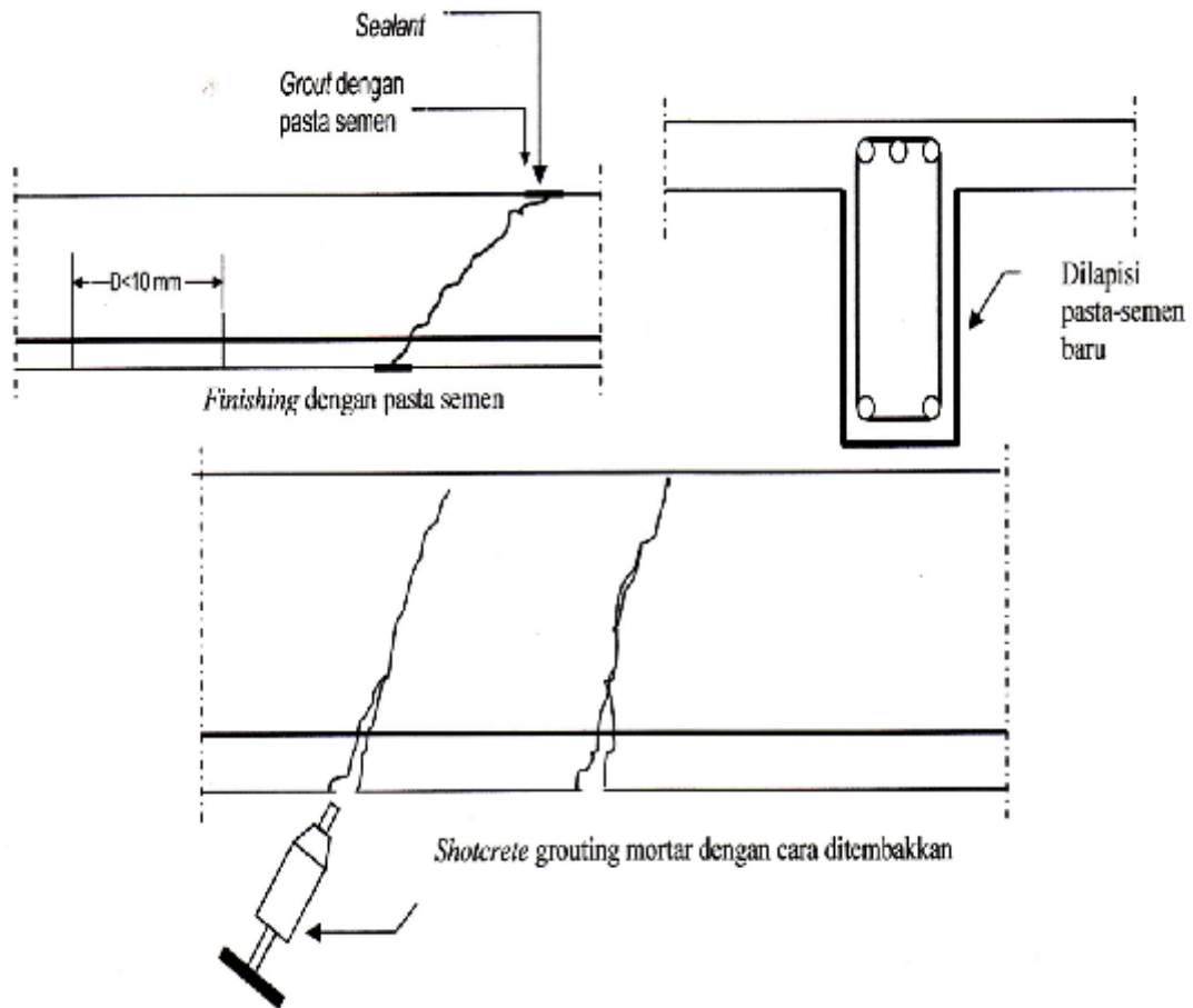
Gambar 3 : Grouting pada plat dan balok lantai
