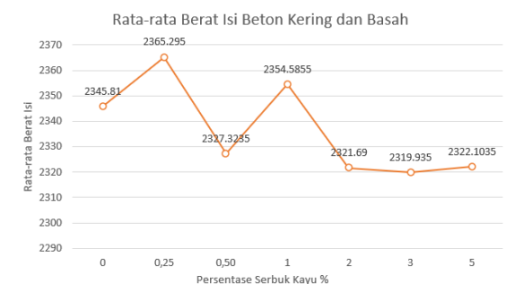
Gambar 6. Grafik rata-rata berat isi beton kering dan basah
