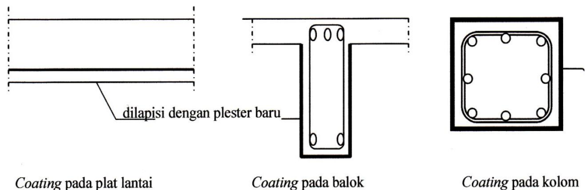
Gambar 2 : Coating pada plat lantai, balok dan kolom
