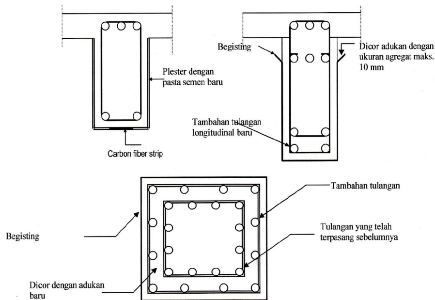
Gambar 4 : Prepacked concrete pada balok dan kolom
