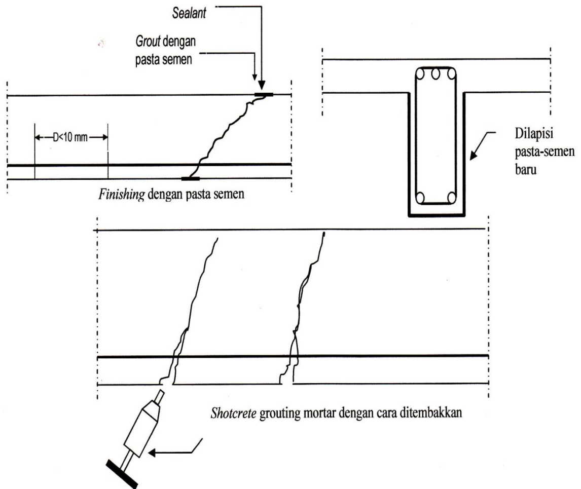
Gambar 3 : Grouting pada plat dan balok lantai
