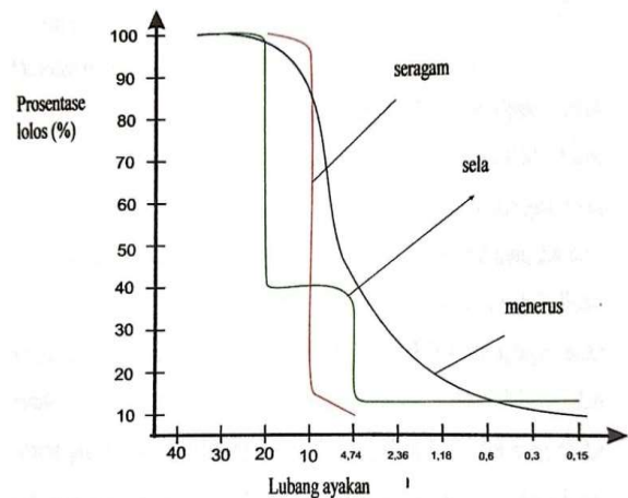
Gambar 2. 1. Jenis gradasi agregat
