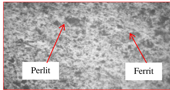
Gambar 15. Struktur mikro media pendingin udara
