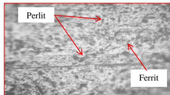
Gambar 13. Struktur mikro media pendingin Oli SAE 40
