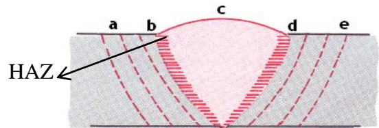
Gambar 6 Titik Pengujian pada HAZ
