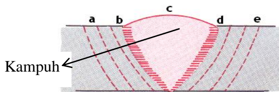
Gambar 8 Titik Pengujian pada HAZ
