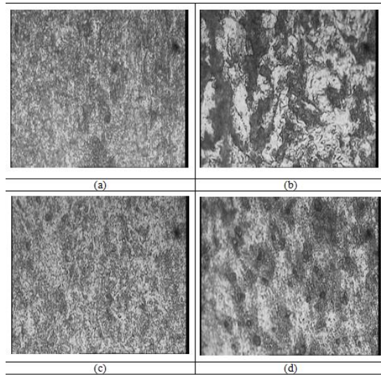
Gambar 7 struktur mikro HAZ pada temperatur (a) PWHT 300°C (B) PWHT 500°C (c) PWHT 700°C (d) tanpa perlakuan
