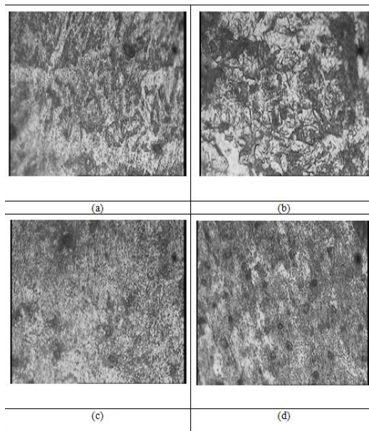
Gambar 9 struktur mikro kampuh las pada temperatur (a) PWHT 300°C (b) PWHT 500°C (c) PWHT 700°C (d) tanpa perlakuan
