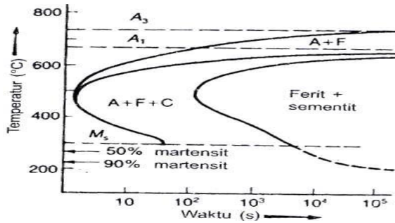
Gambar 3 Diagram TTT
