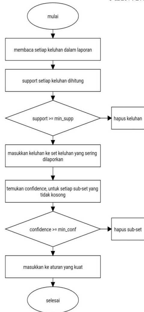
Gambar 5. Flowchart Metode Apriori
