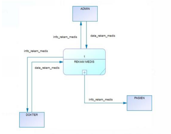
Gambar 3. konteks diagram
