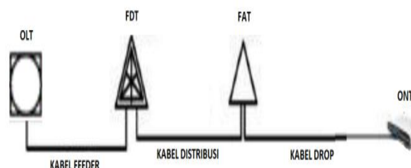
Gbr 1. Struktur jaringan FTTH
