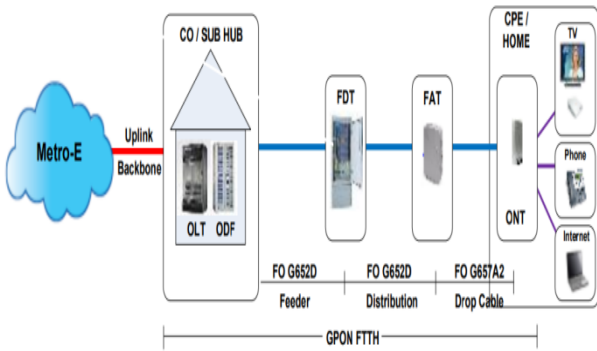
Gbr 2. Struktur jaringan GPON [2]
