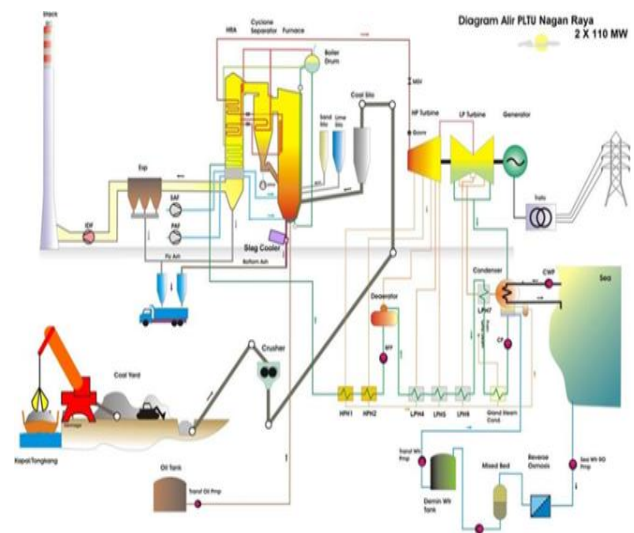
Gbr.5 Diagram Alir PLTU Nagan Raya 2x110 MW
