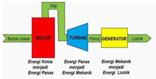
Gbr.1 Proses konversi energi pada PLTU
