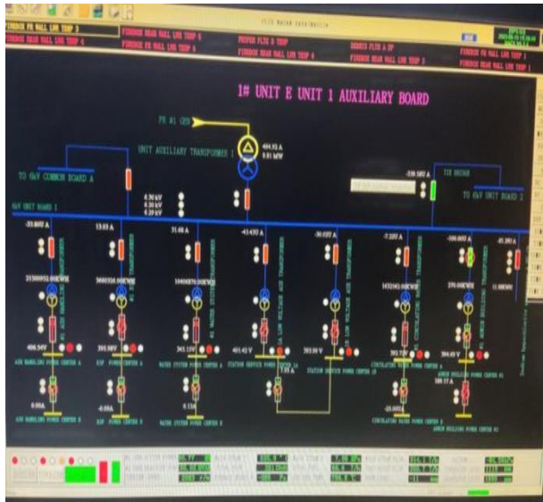
Gbr.6 Single Line Diagram Pembagian Daya Generator
