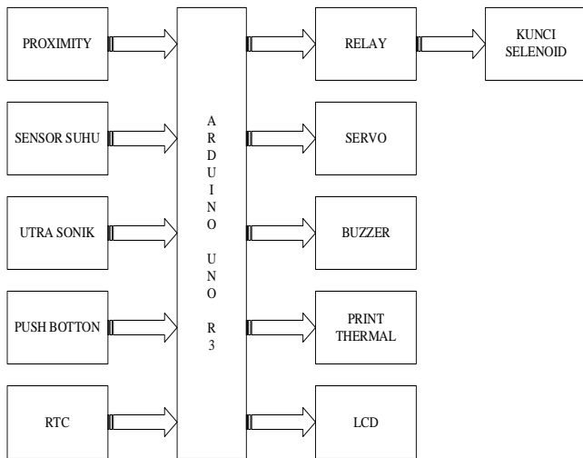
Gambar 7. Blok Diagram Jendela Pintar
