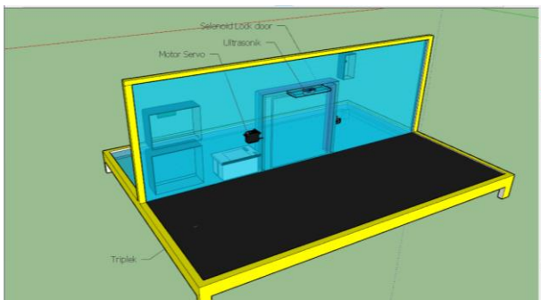
Gambar 10 Tampak belakang alat
