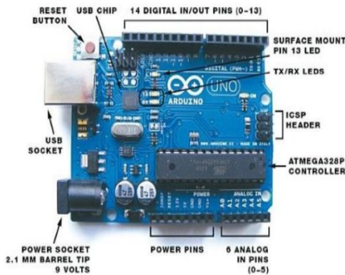
Gambar 1. Arduino Uno R3
