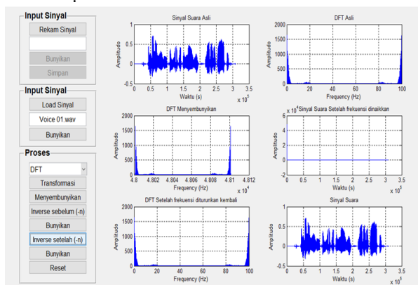
Gambar 7. Menyembunyikan sinyal suara 1 metode DFT
