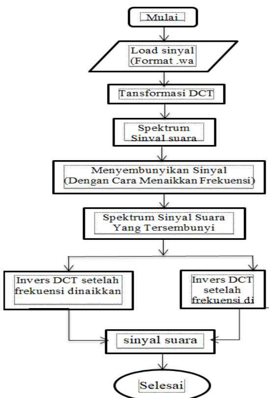
Gambar 4. Flowchart teknik menyembunyikan sinyal suara menggunakan Metode DCT
