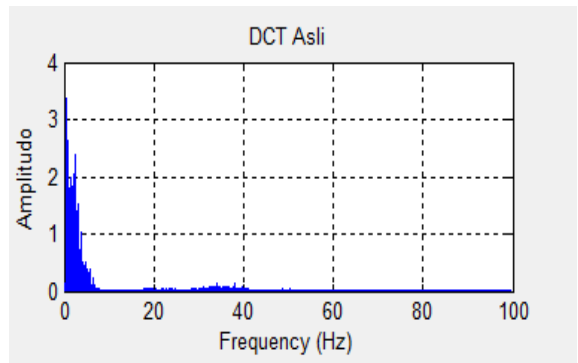
Gambar 13. Transformasi DCT
