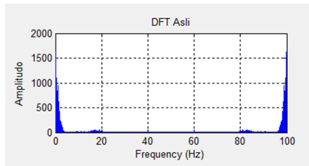
Gambar 8. Transformasi DFT
