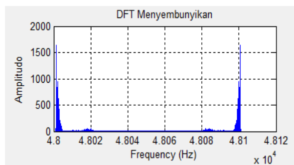
Gambar 9. Menyembunyikan sinyal suara DFT
