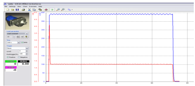
Gambar 13. Data Grafik Hasil Pengujian Relay Berbeban dengan Arus Gangguan 1,3 A
