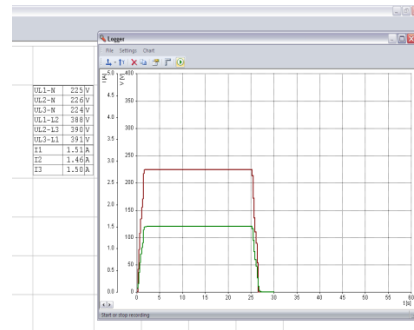
Gambar 11. Karakteristik Relay Arus Lebih Tipe SEL-351A yang Didapatdari Hasil Pengujian Normal Inverse dengan ArusGangguan 1,5 A
