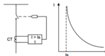
Gambar 1. Karakteristik Tripping relay arus lebih waktu invers.
