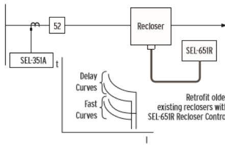
Gambar 6. Mengkoordinasikan Alat Pelindung Arus Berlebih
