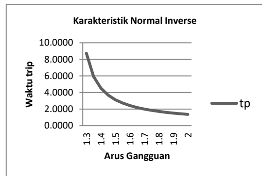
Gambar 12. Karakteristik Relay Arus Lebih Tipe SEL-351A yang didapatdari Hasil Perhitungan Normal Inverse
