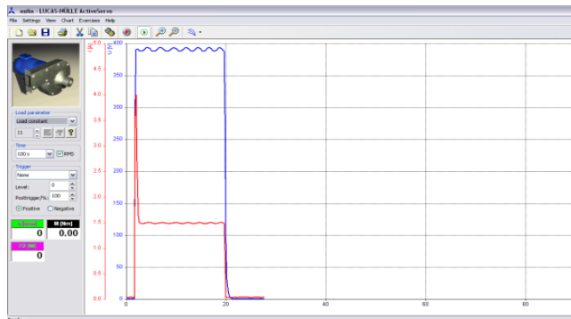
Gambar 14.. Data Grafik Hasil Pengujian Relay Berbeban dengan Arus Gangguan 1,5 A
