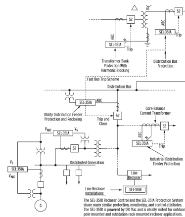
Gambar 5. SEL-351A SistemPerlindungan Terapan Sepanjang Sistem Daya
