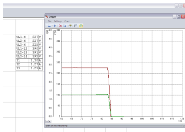
Gambar 7. Karakteristik Relay Arus Lebih Tipe SEL-351A yang Didapatdari Hasil Pengujian Normal Inverse dengan Arus Gangguan 1,30 A
