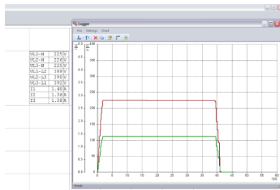
Gambar 9. Karakteristik Relay Arus Lebih Tipe SEL-351A yang didapatdari Hasil Pengujian Normal Inverse dengan Arus Gangguan 1,40 A
