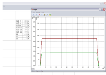
Gambar 8. Karakteristik Relay Arus Lebih Tipe SEL-351A yang Didapatdari Hasil Pengujian Normal Inverse dengan Arus Gangguan 1,35 A
