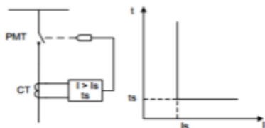
Gambar 3. Karakteristik tripping relay arus lebih waktu definite .
