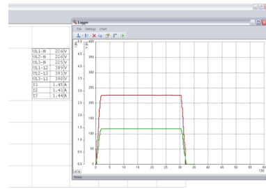
Gambar 10. Karakteristik Relay Arus Lebih Tipe SEL-351A yang didapat dari Hasil Pengujian Normal Inverse dengan ArusGangguan 1,45 A
