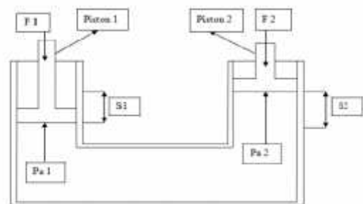
Gambar. 1_Sistem Hidrolik
